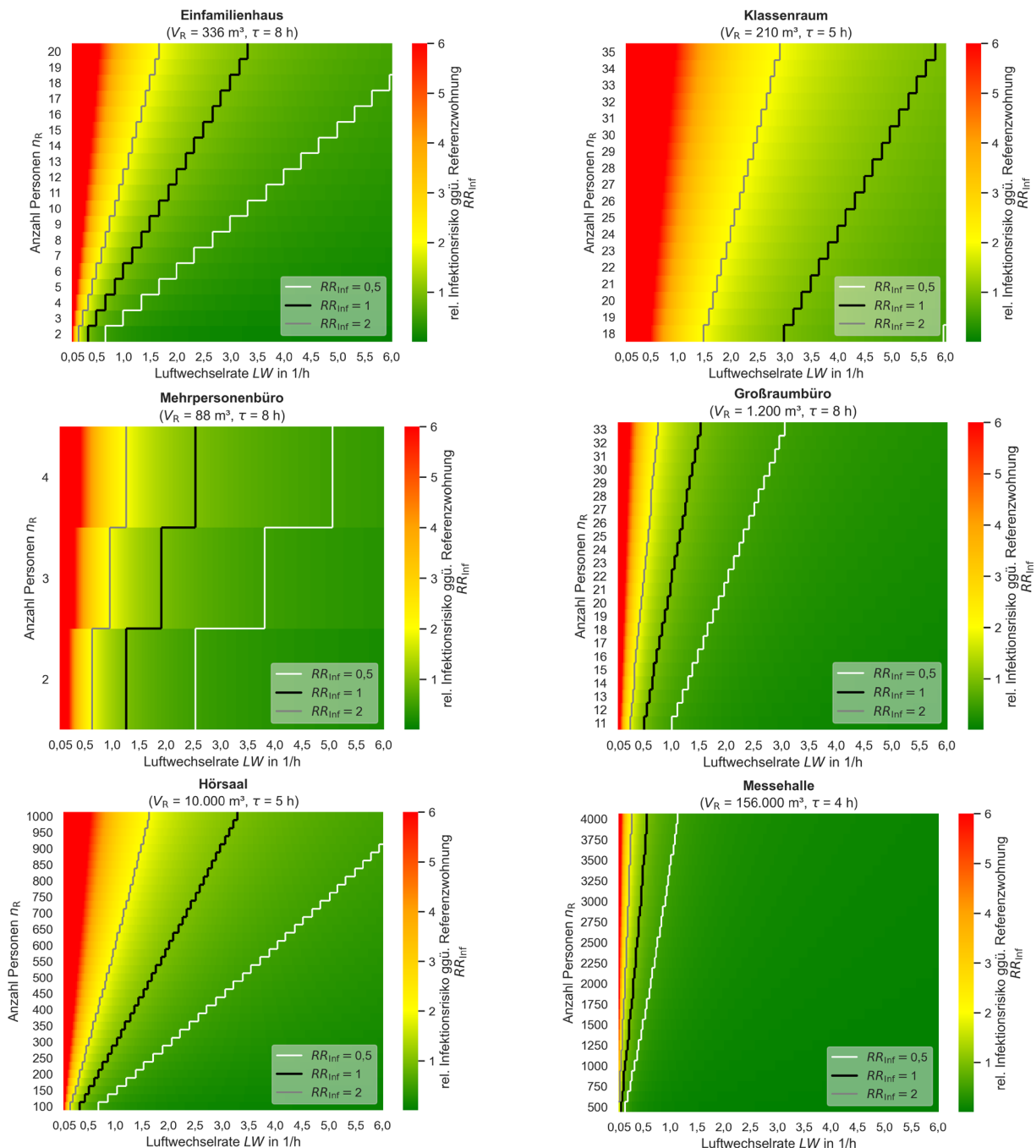
Abbildung 2: Relatives Infektionsrisiko verschiedener immobilier Vergleichsumgebungen gegenüber Referenzwohnung durch Aerosole
