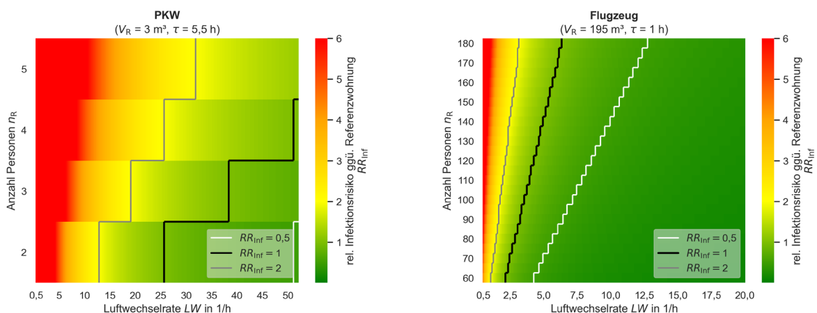
Abbildung 3: Relatives Infektionsrisiko verschiedener mobiler Vergleichsumgebungen gegenüber Referenzwohnung durch Aerosole
